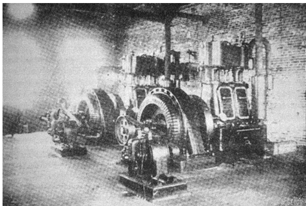
1911年，福州电气股份有限公司新港发电所的发电机组。
