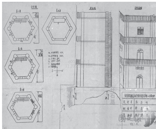
气象台草图—台楼部分（剖面图可见楼基于邻霄台顶的施工方案）（薛纪天提供）
